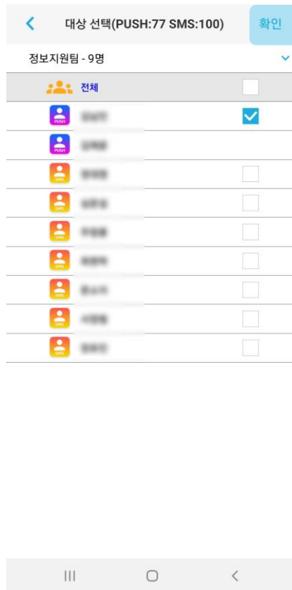
확인 선택
