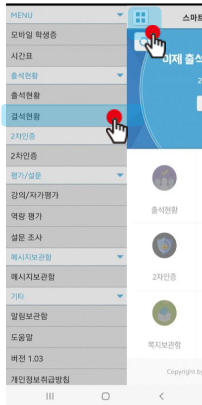
화면 (1)
